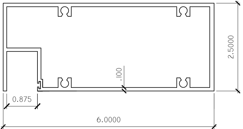
JAMB
